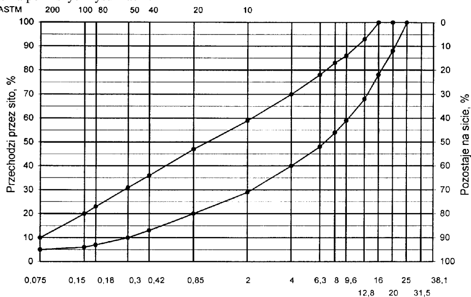
Wymiary oczek sit kwadratowych, mm
